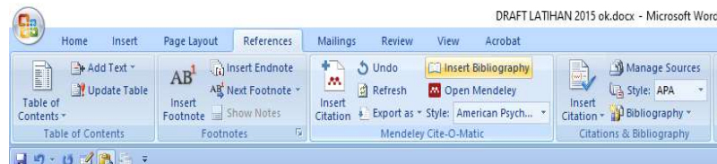
Gambar 8. Menampilkan Bibliography .
